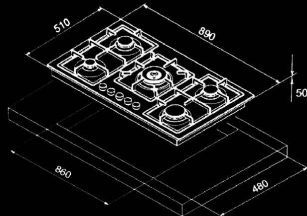
כיריים גז 90 ס"מ IM905
