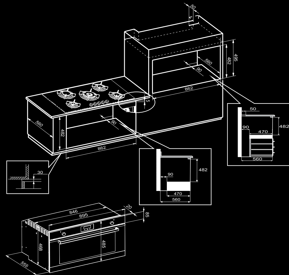
תנור בנוי 90 ס"מ בעיצוב כפרי IM938
