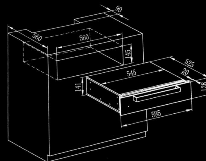
מגירת חימום | WD14 BR
