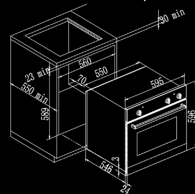
תנור בנוי | IM467 / IM457 / IM767
