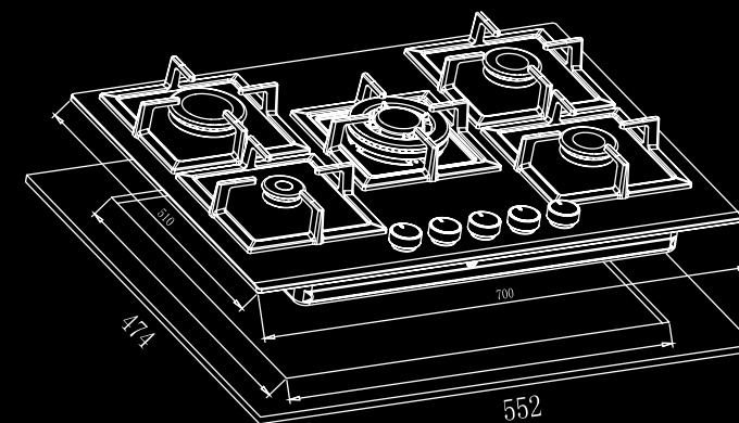
כיריים זכוכית 5 להבות IM7044 / IM7047 / IM7040
