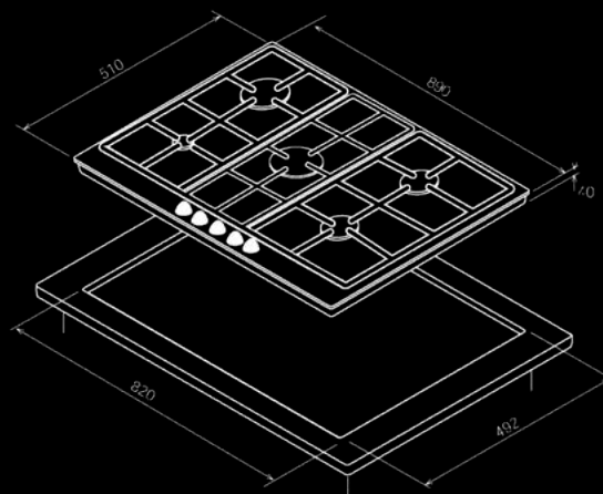
כיריים גז 75 ס"מ IM755
