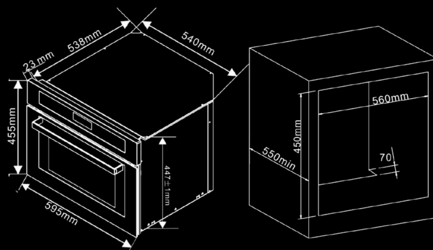
מיקרוגל בנוי | MC316 / MC767
